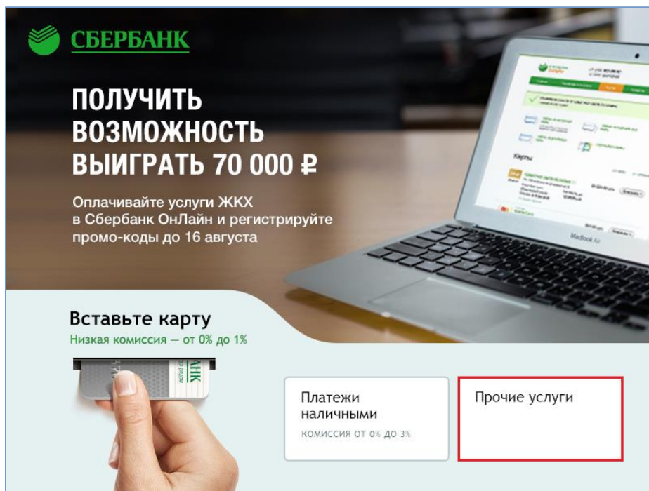
Рис. 1. Начальный экран
